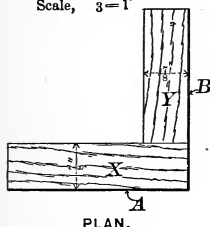
Fig. 199 Scale, 3''=1'
